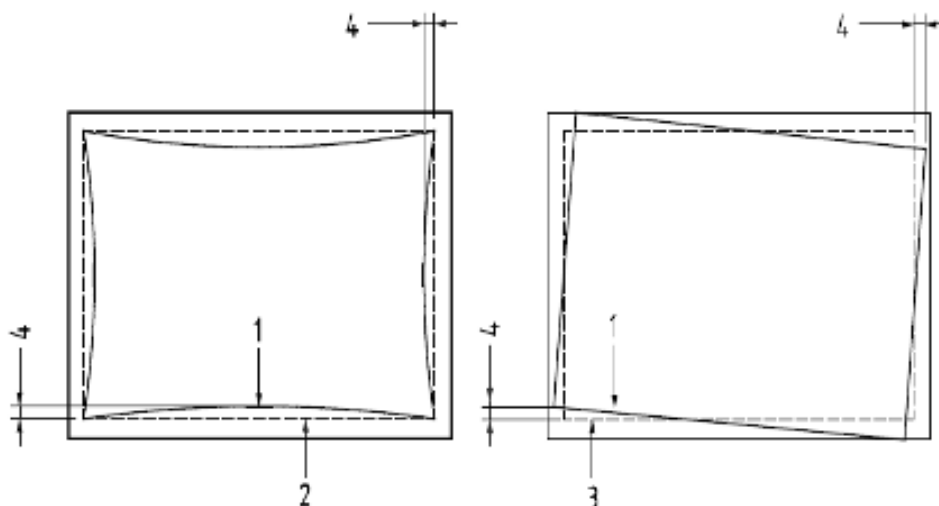
Obrázek č. 2 - tolerance přímosti rámečku
