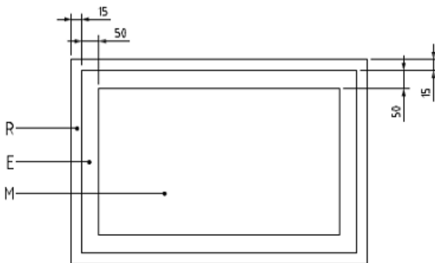
Obrázek 2 – Zóny tabule izolačního skla při posuzování vad
